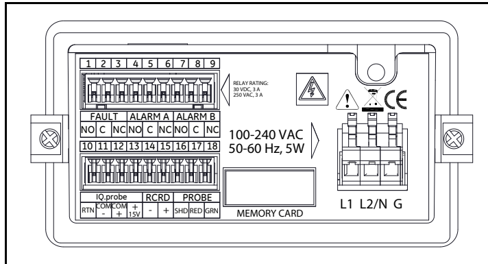
Figure 21: Raccordements électriques (appareils avec bornes d'alimentation CA)
