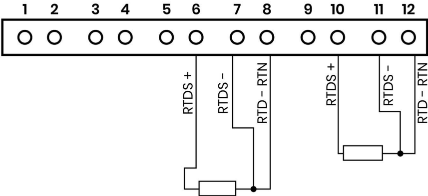
Figura 13: rTD de 3 hilos
