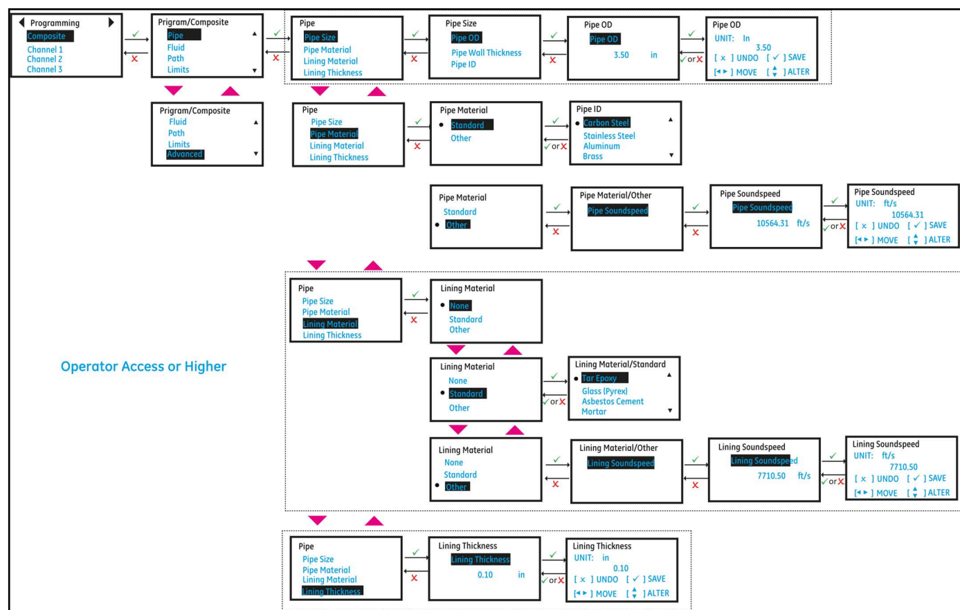
Figura 43: Programación de tuberías
