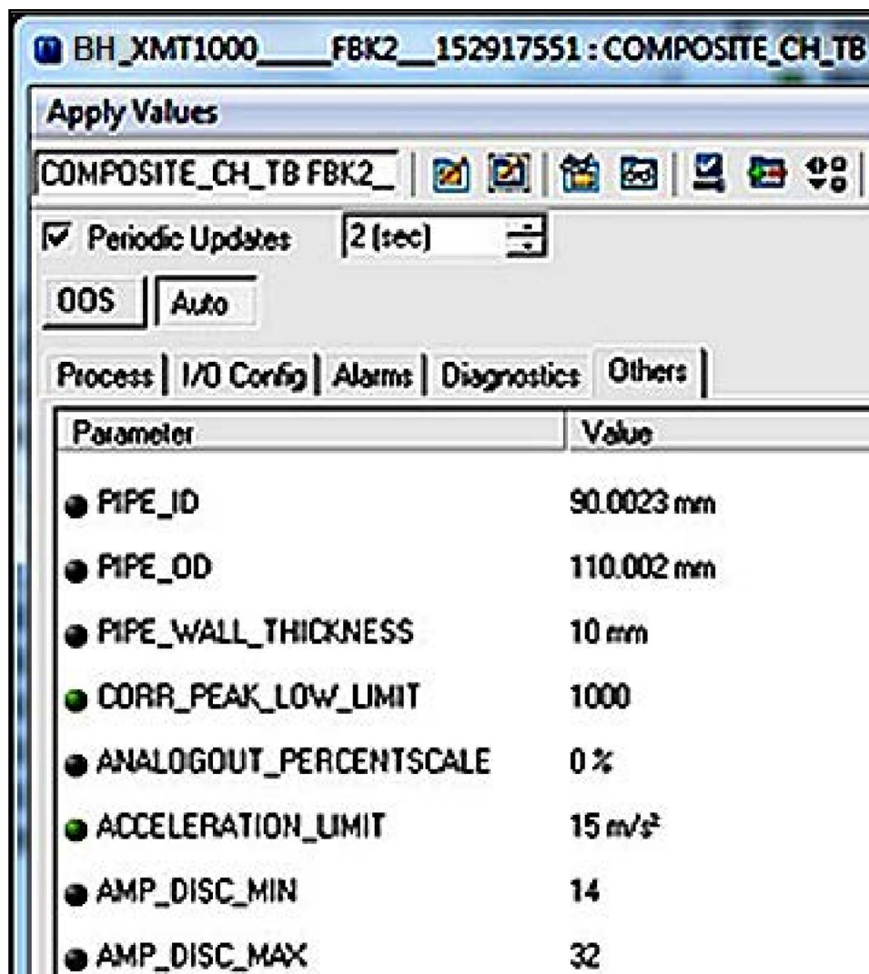
Figura 73: Bloque transductor compuesto
