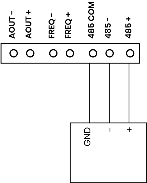
Figura 19: RS-485
