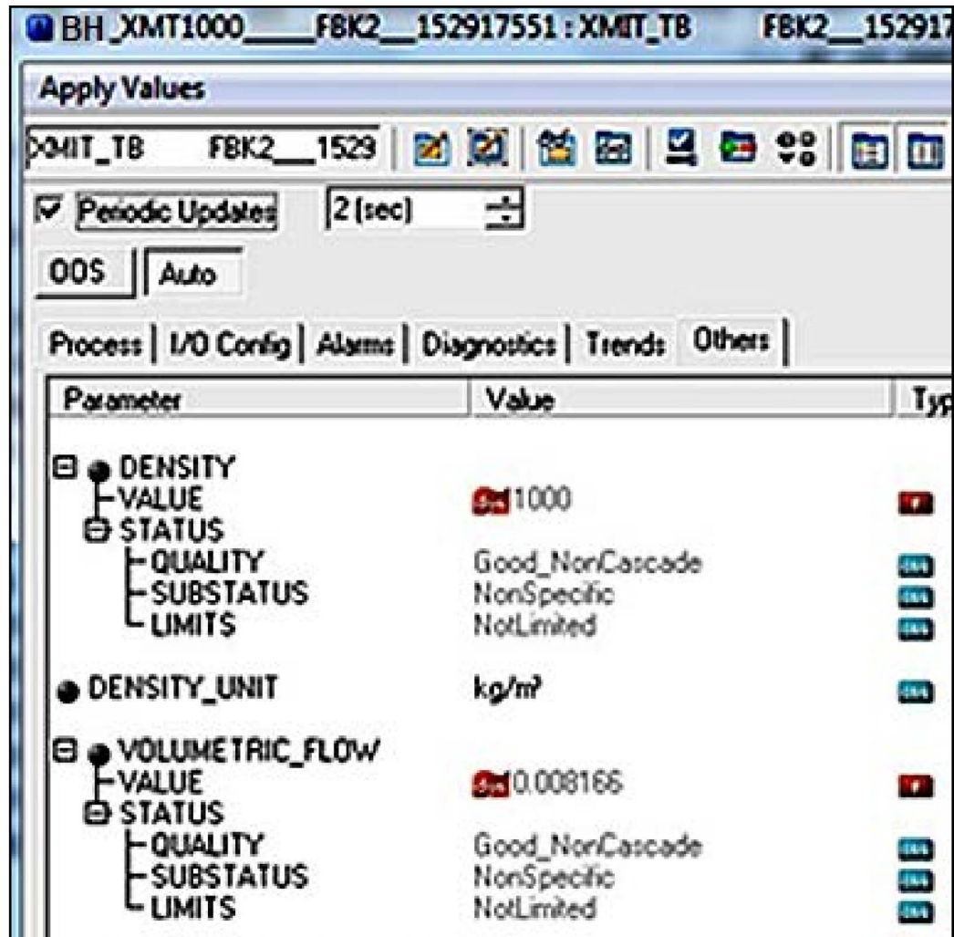
Figura 72: Parámetros y unidades de medida en el bloque transductor XMIT
