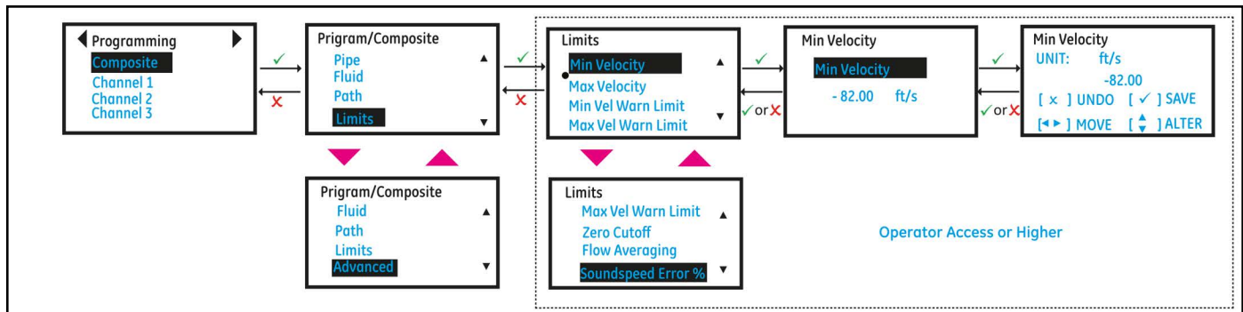
Figura 46: Límites de caudal y diagnóstico
