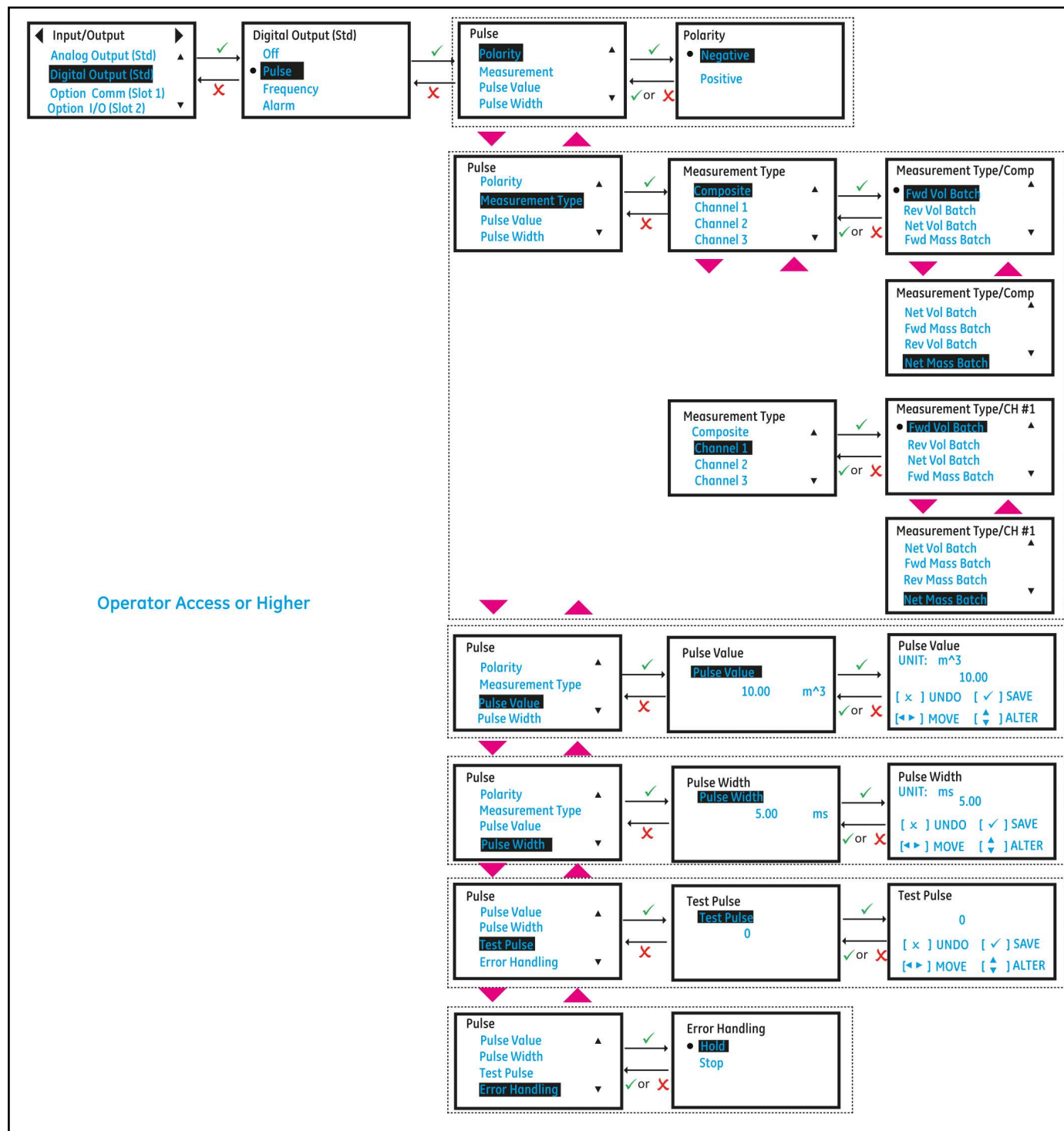
Figura 32: Configuración de la salida de impulsos
