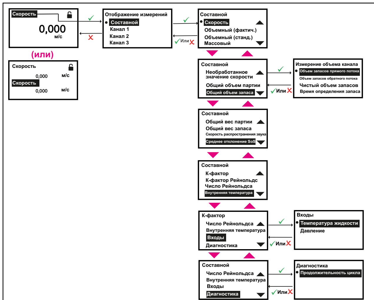
Рисунке 16: Выбор составного измерения для отображения
