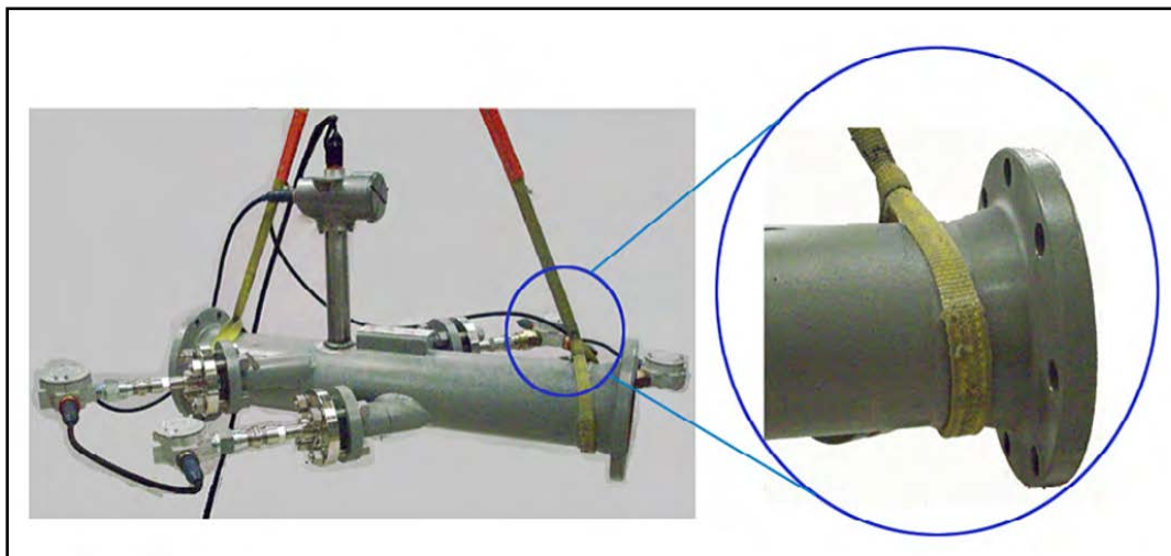
Рисунок 11: Подъем PanaFlow HT
