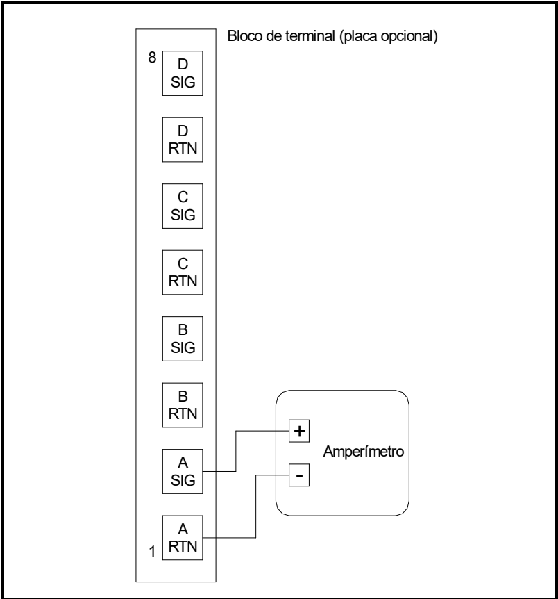
Figura 1-2: Conexão do amperímetro nos Slots 1 ao 6 (Saída A)
