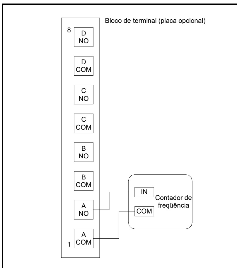
Figura 1-5: Conexões de contador de freqüência
