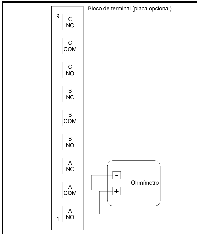
Figura 1-4: Conexões típicas de ohmímetro
