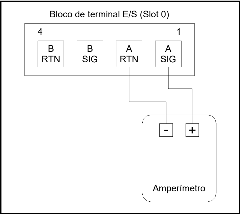
Figura 1-1: Conexão do amperímetro no Slot 0 (Saída A)
