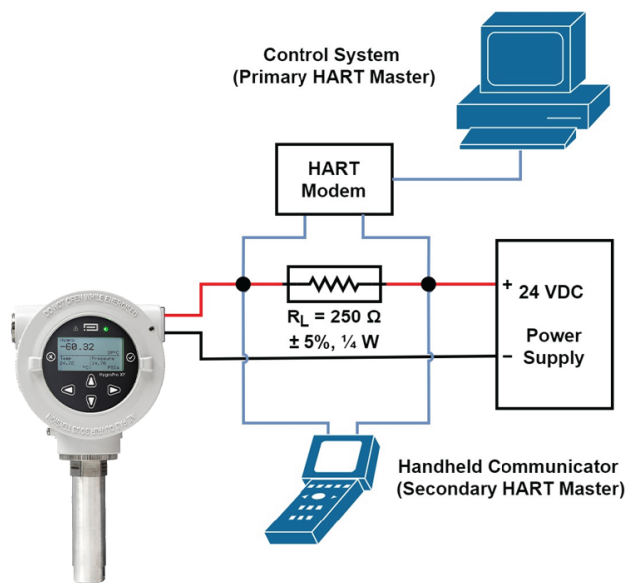
代表的な危険エリアでの設置例であり、アナログ出力デバイスや HARTマスターへの接続を示しています。
