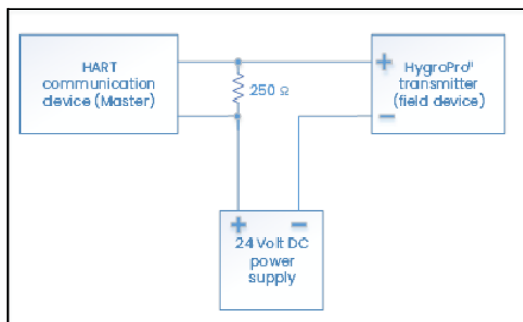
그림 13: HygroPro II 에 마스터 장치를 2개까지 사용할 수 있는 점대점 HART 연결
