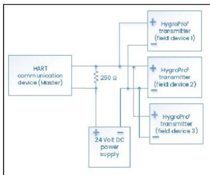
그림 14: 각각 고유한 어드레스가 있는 여러 HygroPro II 송신기가 단일 HART 마스터와 연결되어 있는 멀티드롭 HART 연결
